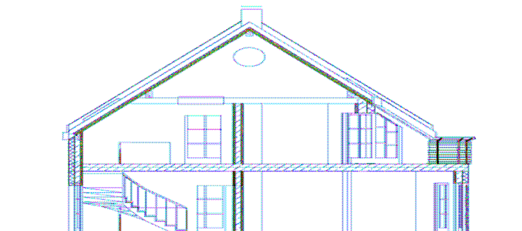
SCHNITT A - A SD 45° KN 1,00m
